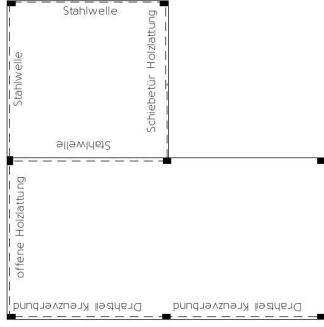
Designo-Einzelcarport mit seitlichem Geräteraum · Ausführung: 1x Designo Grundmodul; 1x Designo Anlehnmodul; 3x Wandelement Stahlwelle; 1x offene Holzlatzung; 2x Drahtseil-Kreuzverbund; 1x Schiebetür offene Holzlatzung
