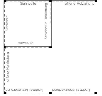
Designo-Doppelcarport mit Geräteraum · Ausführung: 2x zusätzliche System-Stütze; 4x Wandelement Flachwand mit Spritzputz; 1x offene Holzlatzung; 1x Drehtür Stahlwelle
