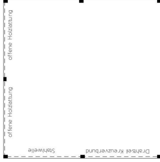
Designo-Doppelcarport · Ausführung: 1x zusätzliche System-Stütze; 2x Wandelement offene Holzlatzung; 1x Stahlwelle; 1x Drahtseilkreuzverbund
